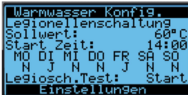
Abbildung 6: Beispieleinstellung Legionellenschaltung
